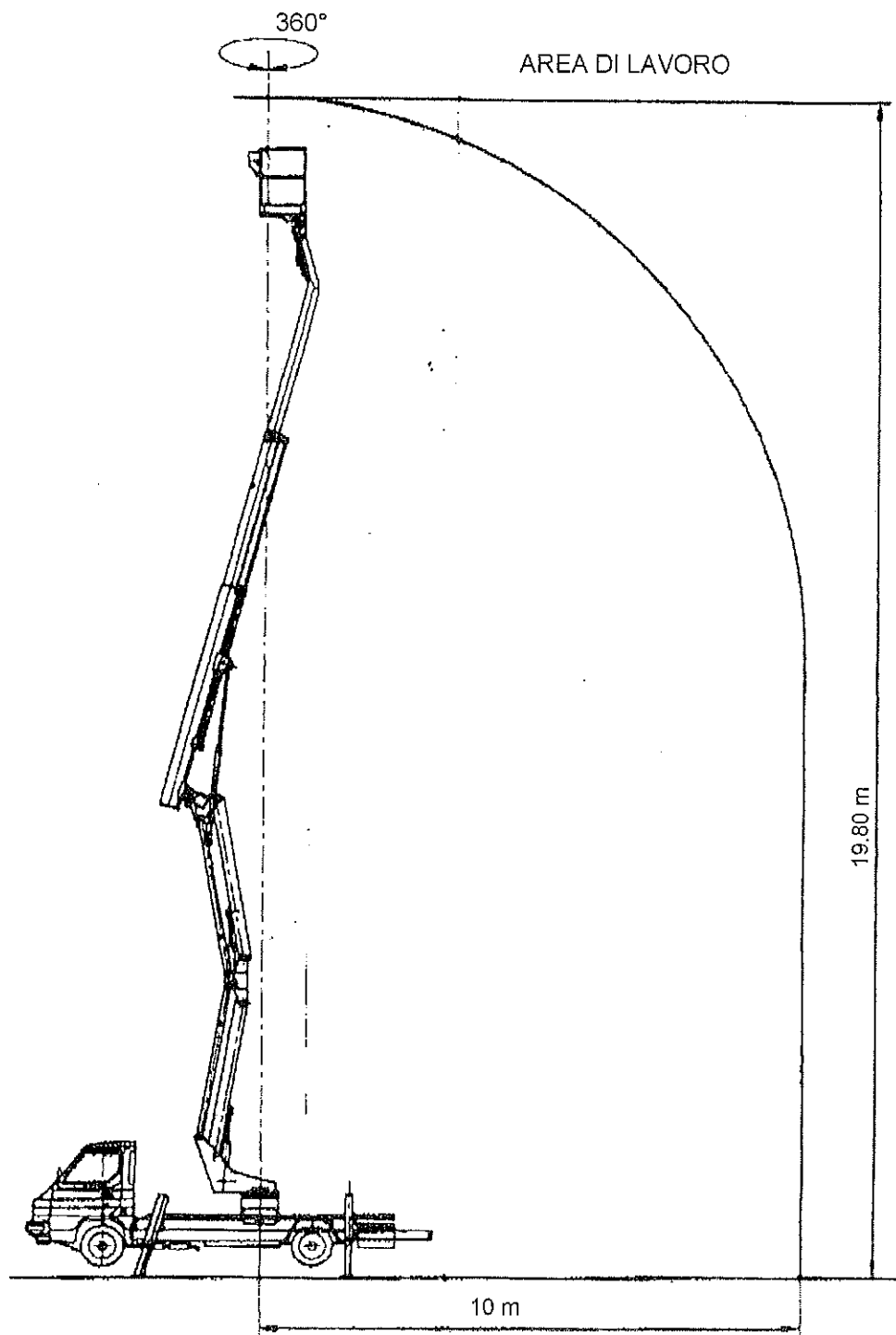
AUTOTELAIO NISSAN TRADE 100 PASSO 3400 MM
